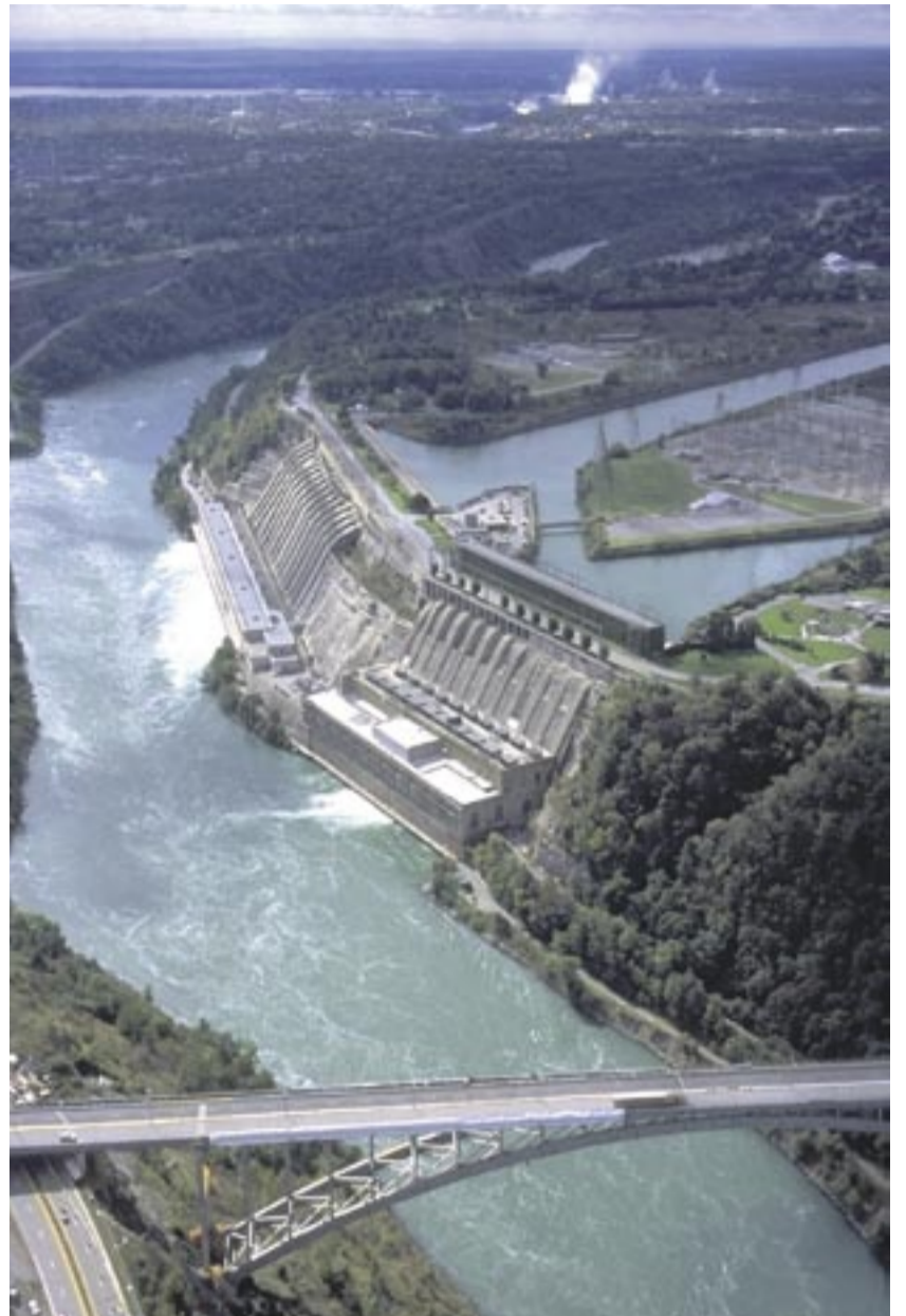
Zusätzlich 500 Kubikmeter Wasser pro Sekunde aus dem Niagara River müssen über einen neu zu errichtenden Stollen zum vorhandenen Krafthaus geleitet werden.
